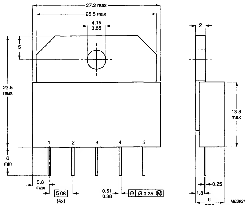
SOT348
