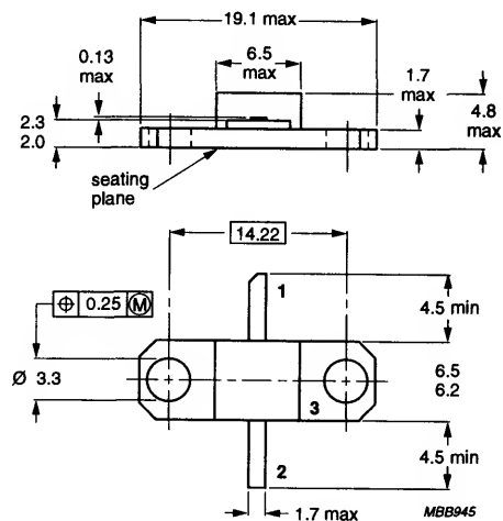
FO229
