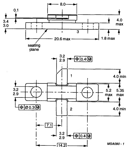
FO83
