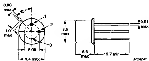
TO-39(b)
