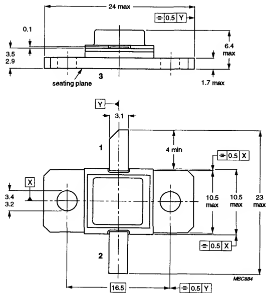
FO57D
