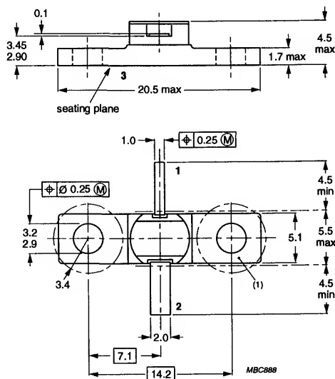
FO41B
