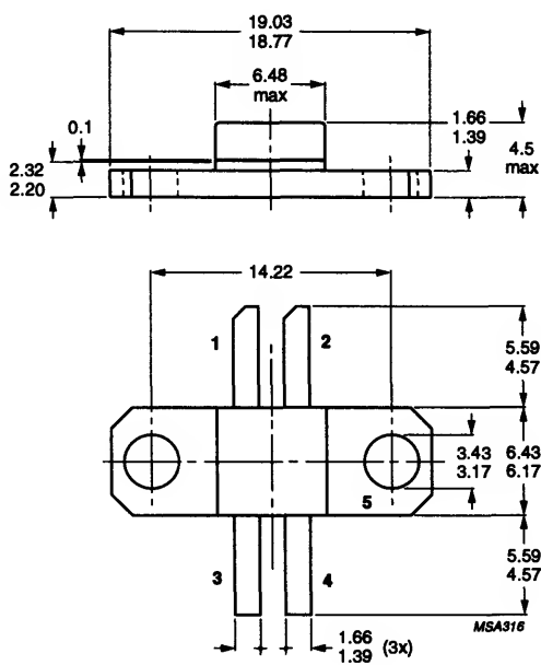
SOT324
