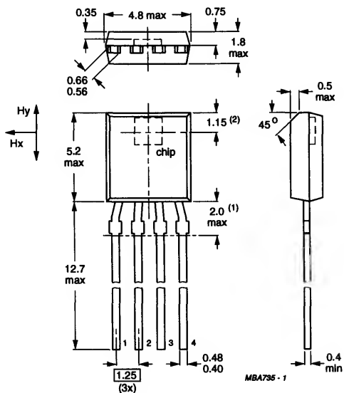
SOT195
