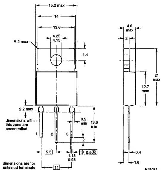
SOT93
