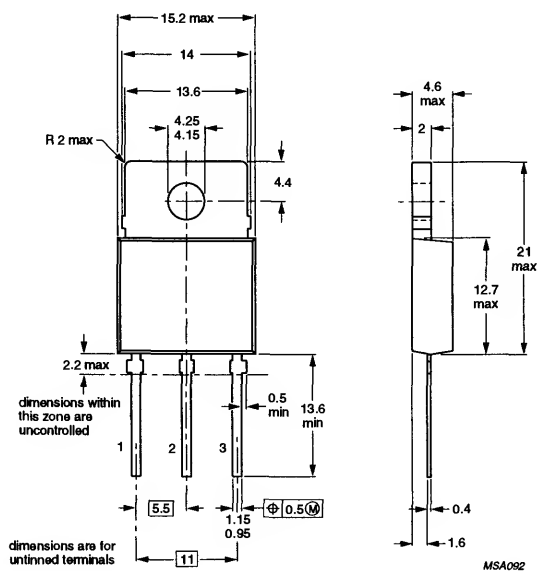
SOT93A
